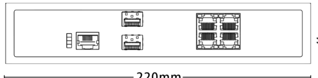
220mm 前视图
